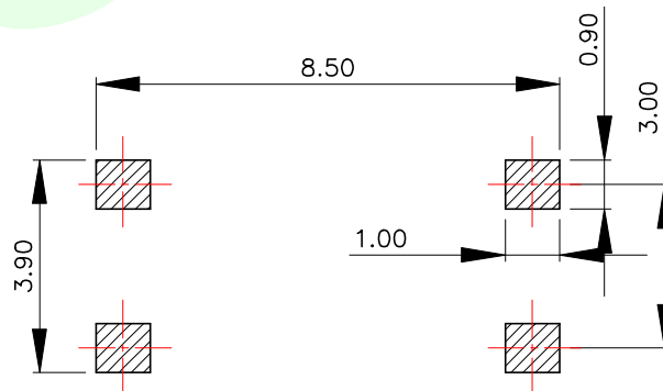
PCB. 焊接图
